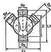
Typ II - pravý i levý přítok
