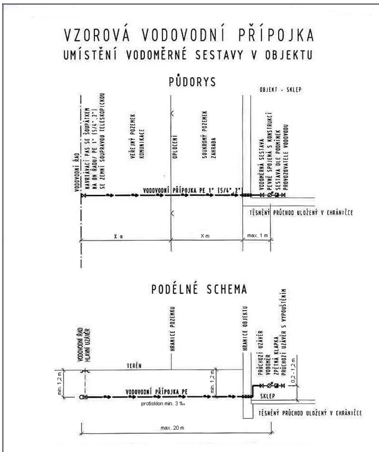
V1 – Vzorová vodovodní přípojka, umístění vodoměrné sestavy v objektu
